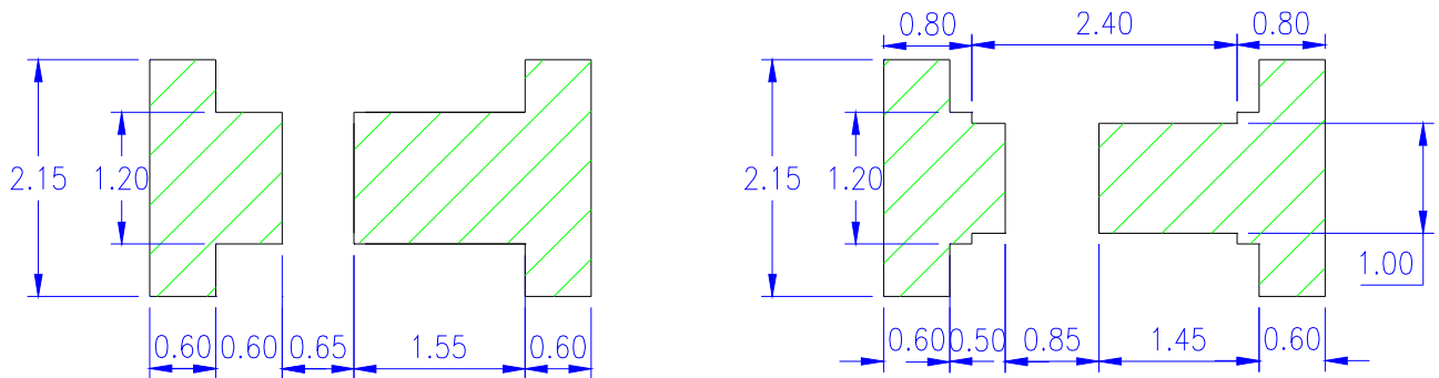
焊盘图
