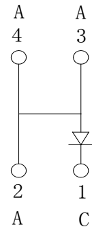
Fig. 1-4 Polarity极性
