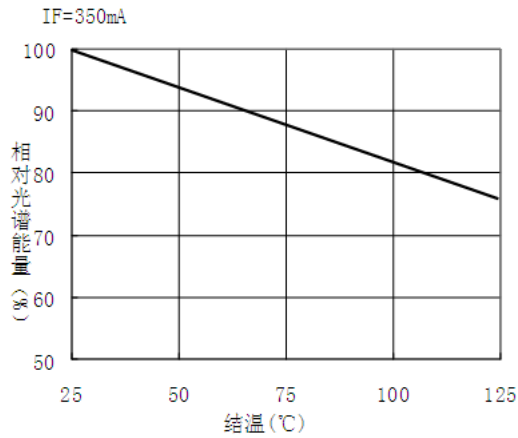
■ 结温——相对光谱能量特性曲线图
