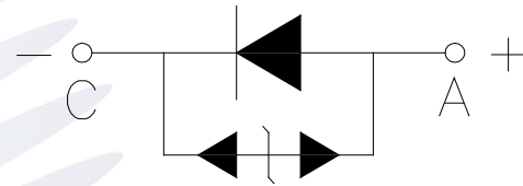
Fig.1-4 Polarity 极性
