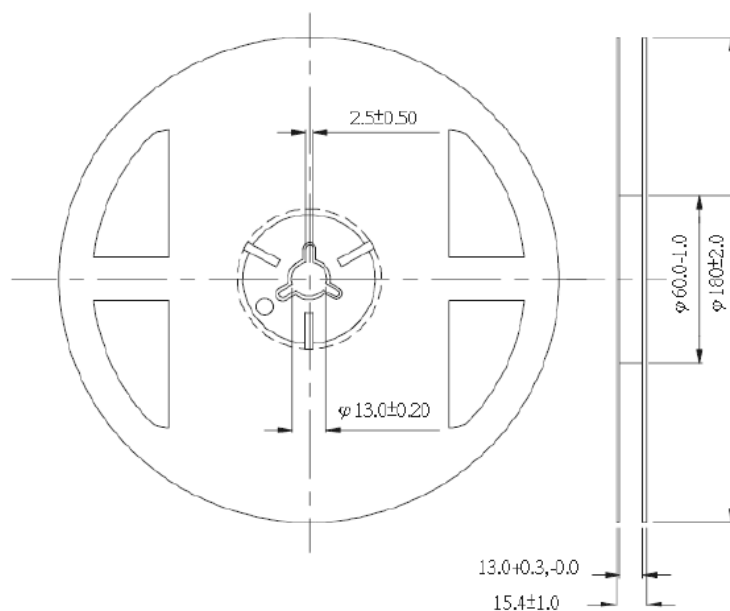
Reel Dimensions
