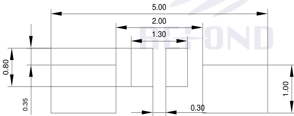
Fig.1-3 Bottom view 背面视图
