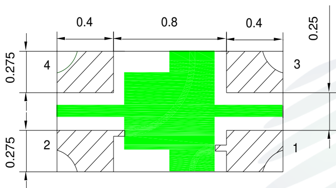
Fig.1-3 Bottom view 背面视图
