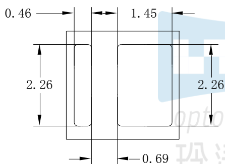
Fig.1-3 Bottom view 背面视图
