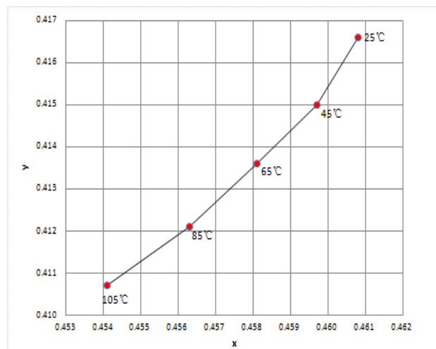
Fig 8. Ta vs. CIE x, y Shift
