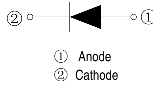
Fig.1-2 Polarity 极性
