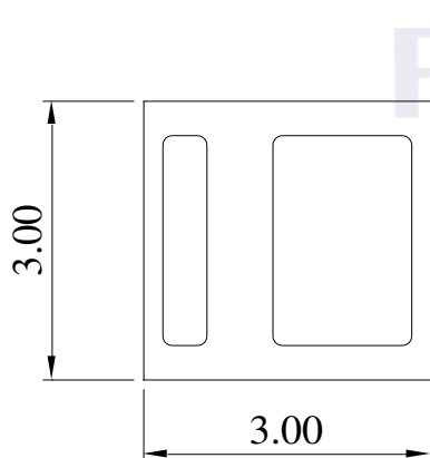
Fig.1-4 Bottom view 背面视图
