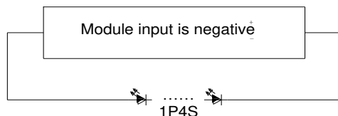
Fig.2-2ED Module connection 模组电性图
