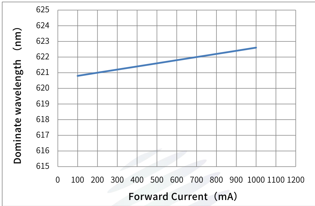
Fig. 1-12 Forward current vs.Dominate wavelength 正向电流与主波长特性曲线(Ts=25°C)
