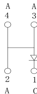
Fig. 1-4 Polarity 极性
