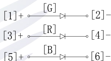
Fig. 1-4 Polarity 极性
