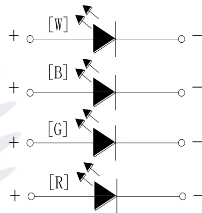
Fig.1-4 Polarity 极性
