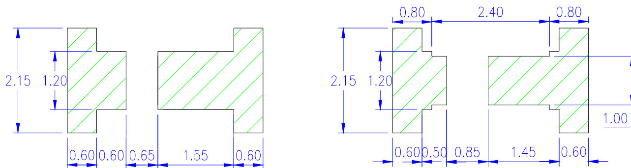
焊盘图
