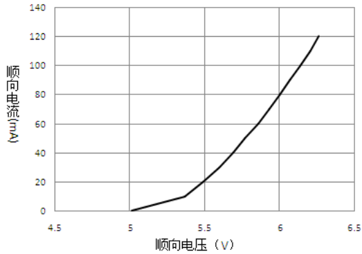
■ 顺向电压——顺向电流曲线图
