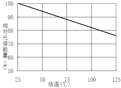
■ 结温——相对光谱能量特性曲线图 IF=80mA
