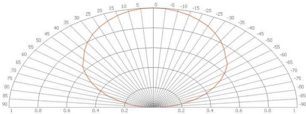
■ 发光角度图
