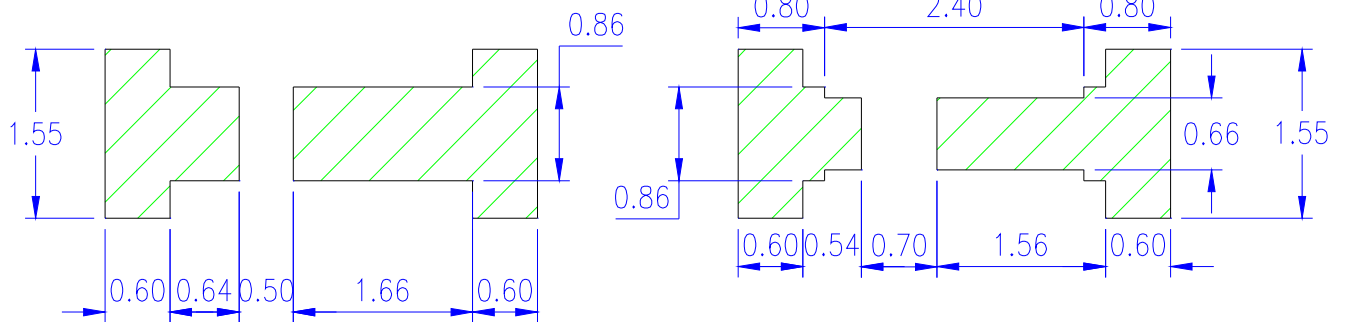
焊盘图
