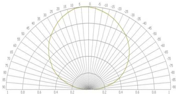
■ 发光角度图
