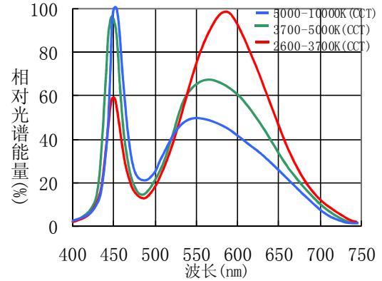
■ 相对光谱能量曲线图
