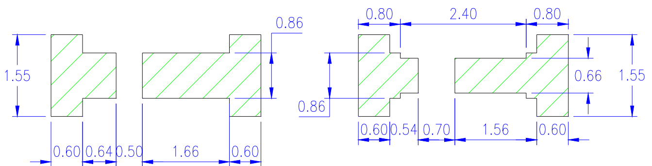
焊盘图
