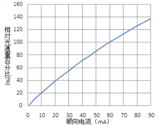
■ 顺向电流——相对光通量曲线图
