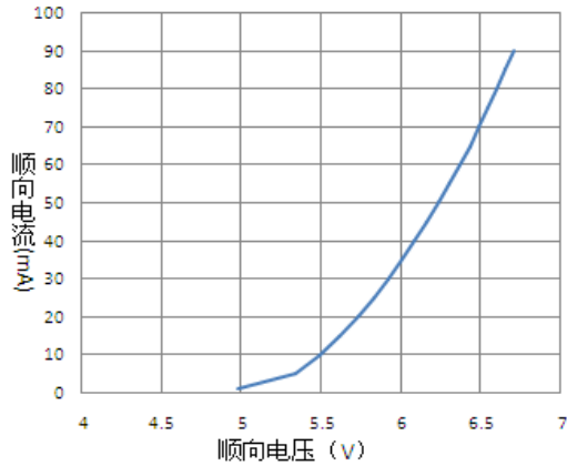
■ 顺向电压——顺向电流曲线图
