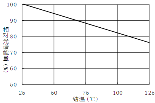
■ 结温——相对光谱能量特性曲线图
