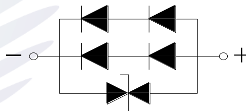
Fig.1-4 Polarity 极性
