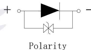
Fig.1-4 Polarity 极性
