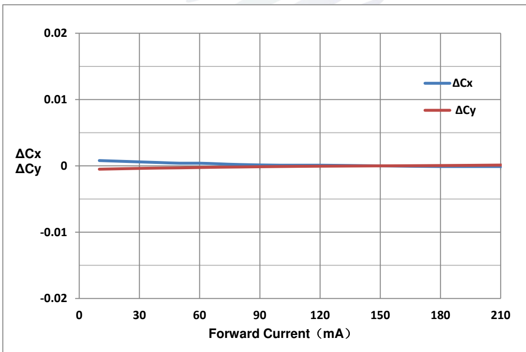
Fig. 1-17 Chromaticity Coordinate Shift Vs Forward Current (Amber) 色坐标偏移与正向电流特性曲线 (琥珀光)
