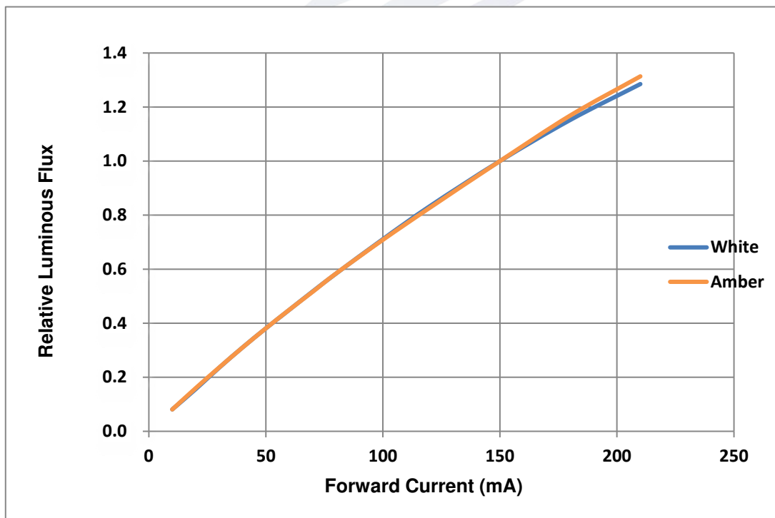
Fig. 1-9 Forward Current Vs Relative Luminous Flux 正向电流与相对光通量特性曲线
