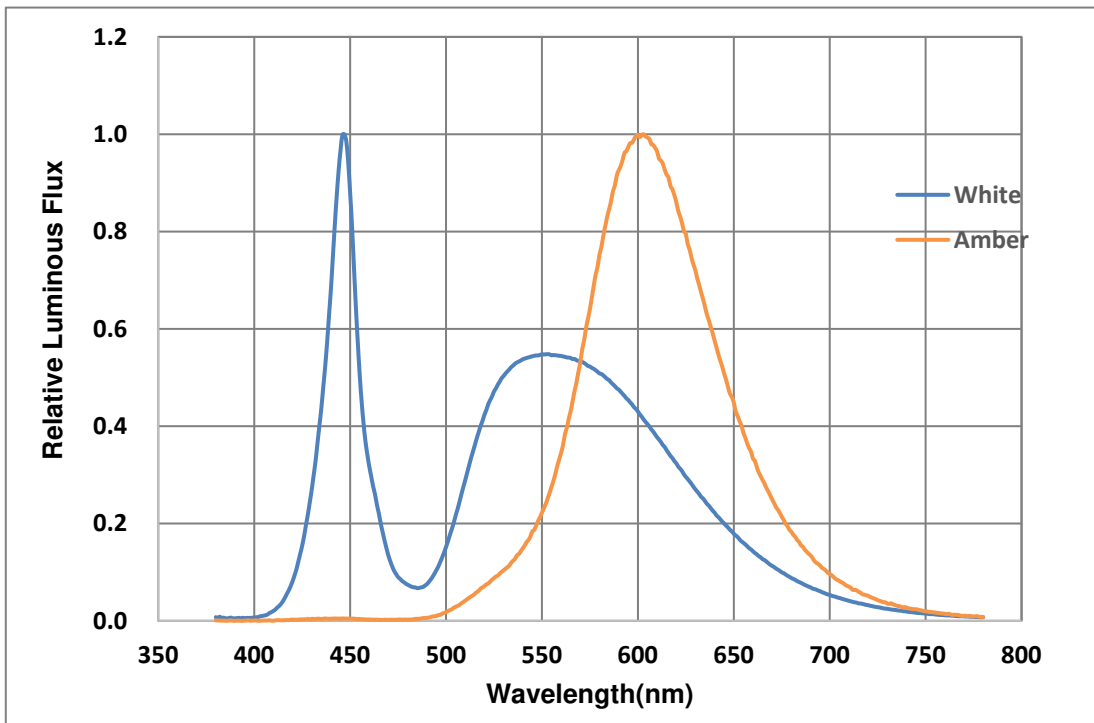
Fig. 1-18 Spectrum Distribution 光谱分布特性曲线
