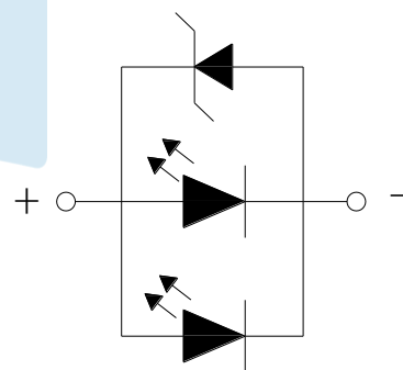
Fig.1-4 Polarity 极性
