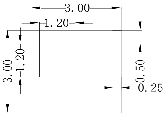
Fig.1-1 Top View 正面视图
