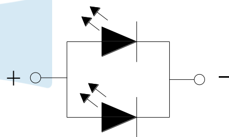
Fig.1-4 Polarity 极性
