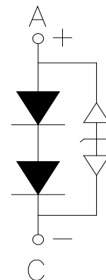
Fig.1-4 Polarity 极性
