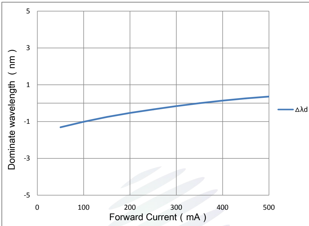
Fig. 1-12 Forward current vs.Dominate wavelength 主波长与正向电流特性曲线
